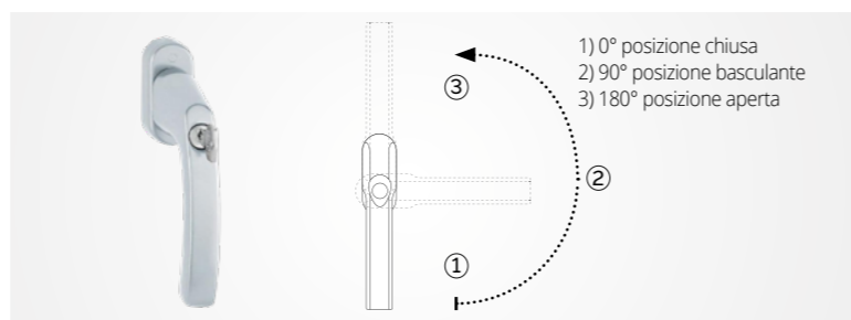
FERRAMENTA TBT (TILT BEFORE TURN) inclinare prima dell'apertura - protezione con chiave contro l'apertura totale della finestra
